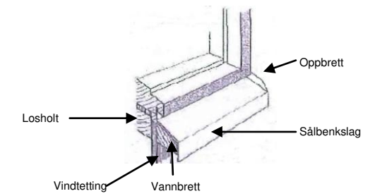
Plassering av sålbenkslag
