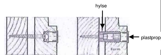
Innfesting med feste- og justeringshylser
