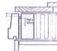
Tetting med fugeskum
