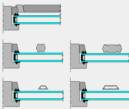
↑ Utenpåliggende sprosser
