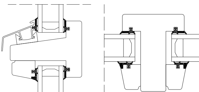
Horisontale sprosser
